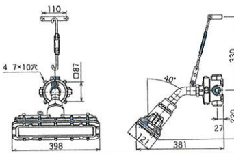
寸法
