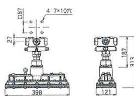
寸法
