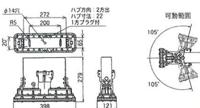
寸法
