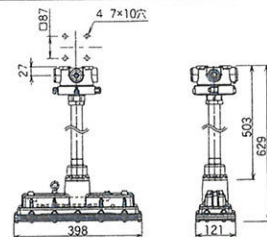
寸法
