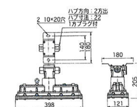
寸法
